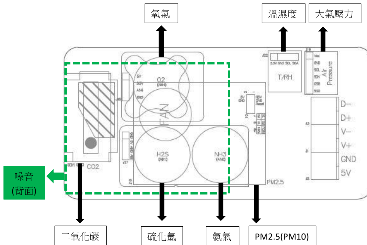
OA4 V1.1 感測器位置圖
