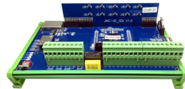
鋁軌型
